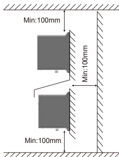
图3 上下安装
