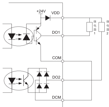
1. 110KW 以上 - 使用内部电源
