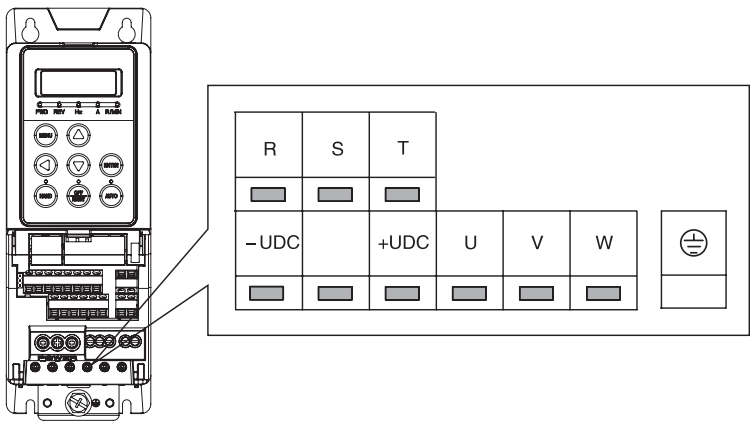
SP1~SP4 机箱主回路端子示意图
