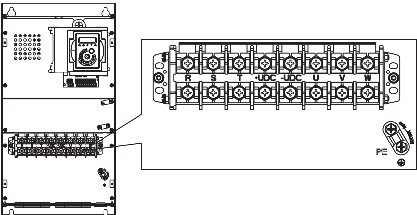
SP5~SP7 机箱主回路端子示意图
