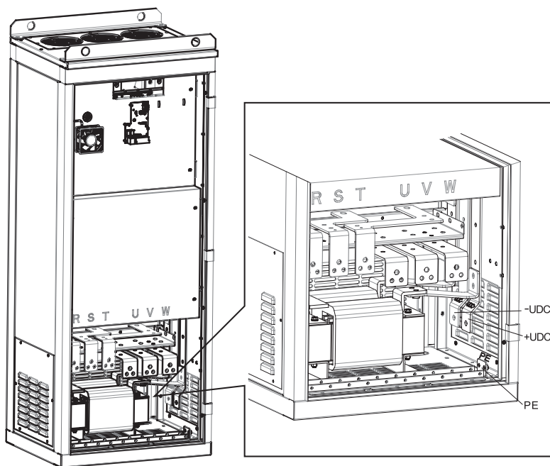
SP10 机箱主回路端子示意图
