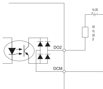
2. 110KW 以上 - DO2 使用外部电源隔离
