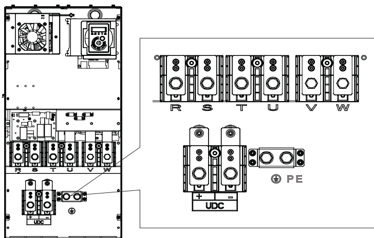
SP8~SP9 机箱主回路端子示意图
