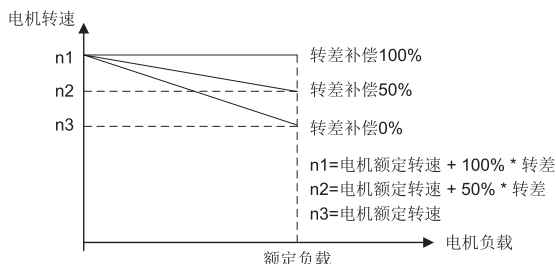
电动时的转差补偿
